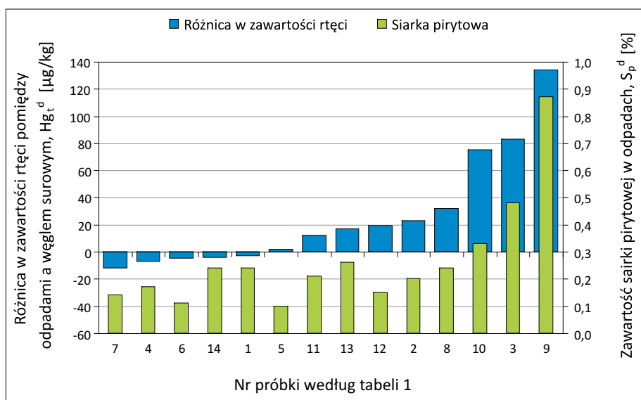
Rys. 6. Różnica zawartości rtęci w odpadach i węglach surowych na tle zawartości siarki pirytowej w odpadach
