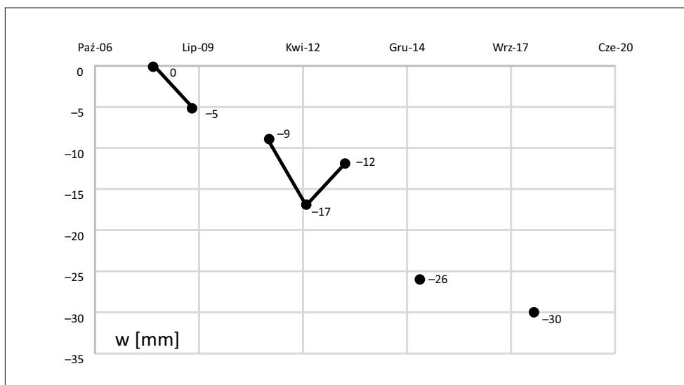
Rys. 3. Obniżenia w czasie repera zastabilizowanego na budynku – w
