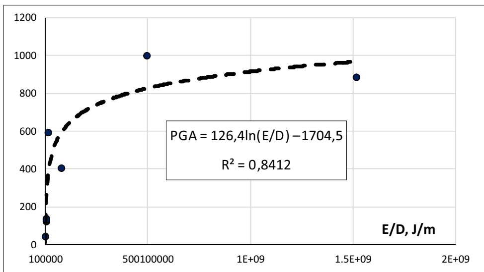
Rys. 9. Wyniki pomiarów PGA dla wstrząsów o największych wartościach energii i aproksymująca je funkcja
